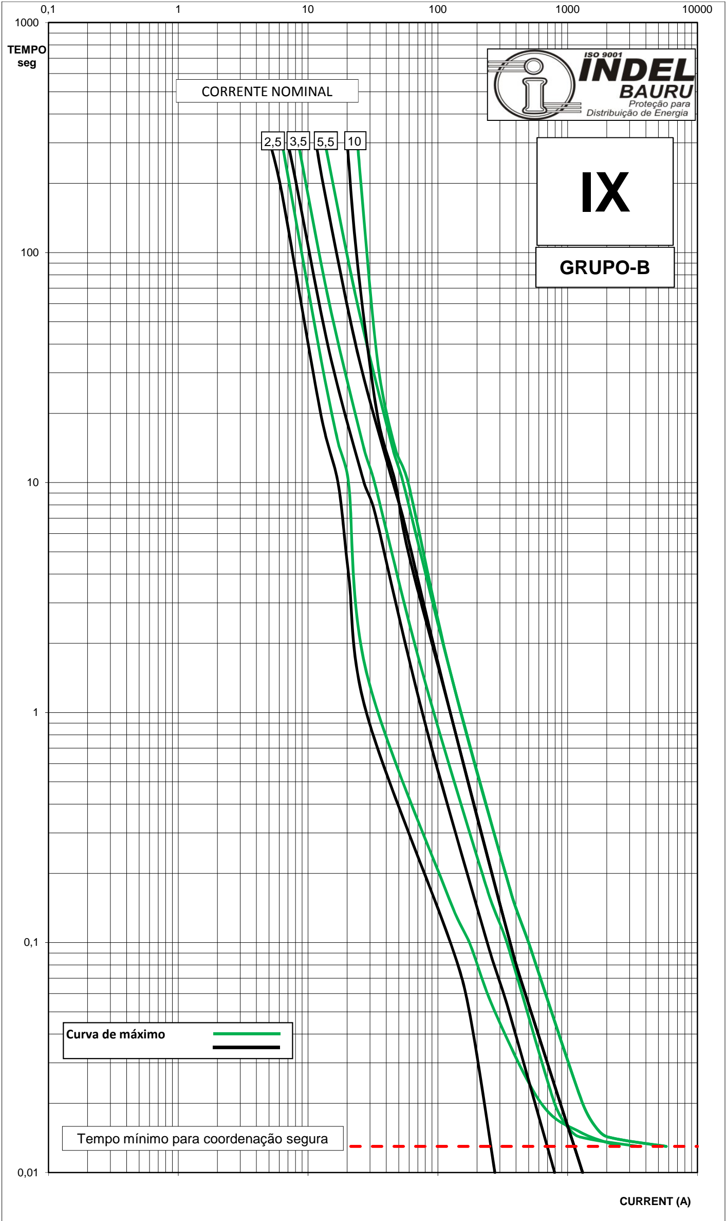
CURVAS CARACTERÍSTICAS DE FUSÃO TEMPO X CORRENTE TIPO "IX" - EM CONFORMIDADE COM A NORMA ANSI C34.42-1996 DATA: 07/10
